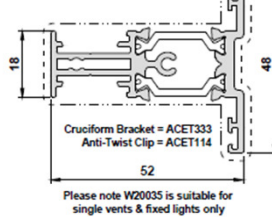
W20135 Door Transom
