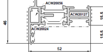
W20027 Door Sash
