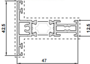
W20135 Door Transom
