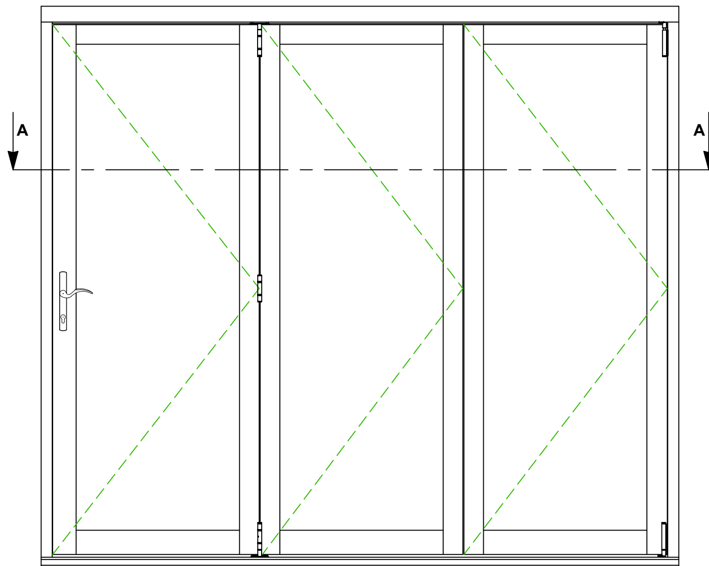
303 DOOR CONFIGURATION
