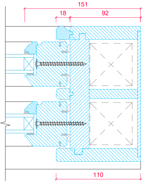
RH JAMB SECTION
