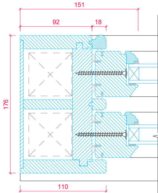
LH JAMB SECTION
