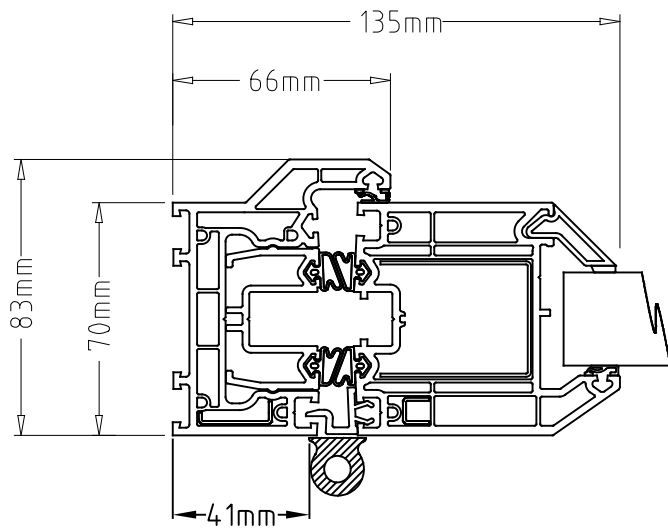
HINGE JAMB
