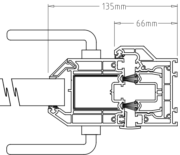
LOCK JAMB
