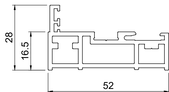
60847 INTERNAL DOOR OUTER FRAME
