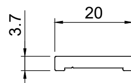
60053 20mm ASTRAGAL BAR
