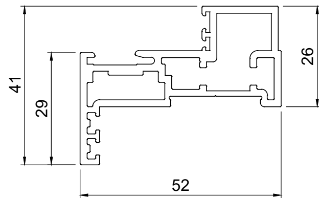
60849 INTERNAL DOOR SASH
