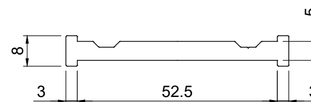
60054 5mm COUPLER
