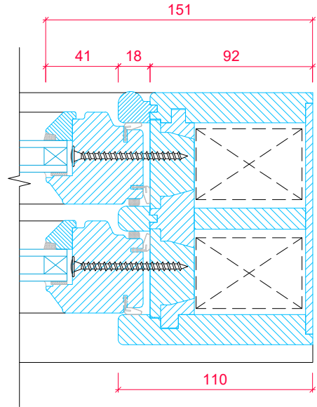
RH JAMB SECTION
