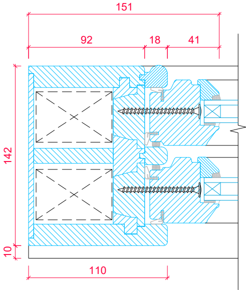
LH JAMB SECTION
